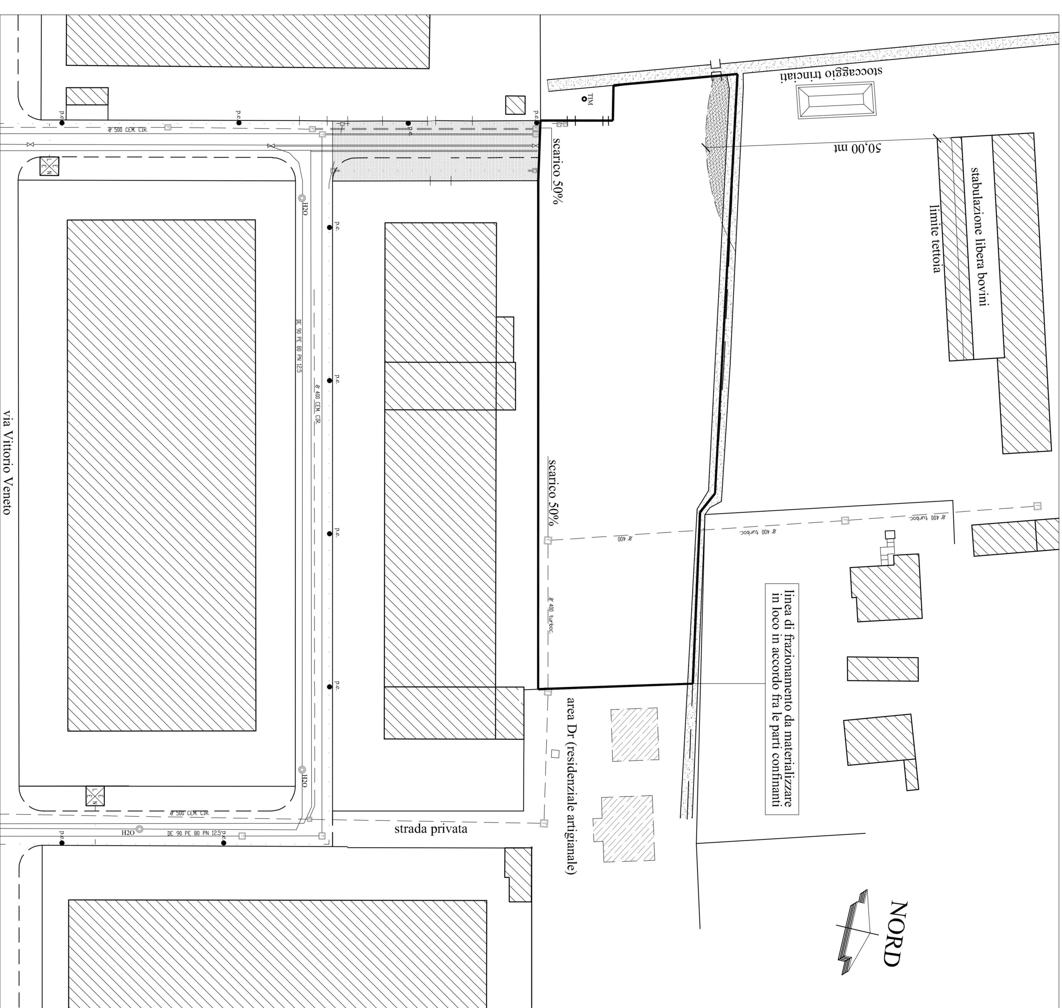
OPERE DI URBANIZZAZIONE 1:500
